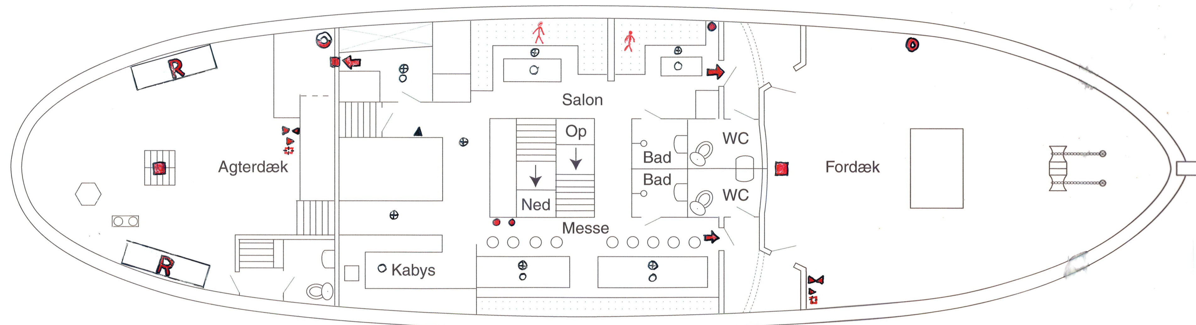
Over dæk er Kisaq indrettet med en rummelig salon og messe
